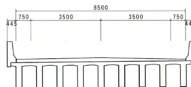
橋梁区間標準横断面図
