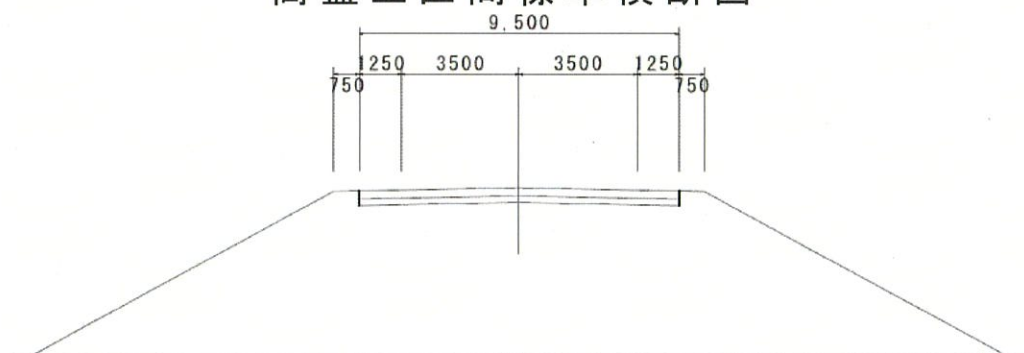
高盛土区間標準横断面図
