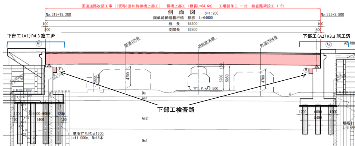
側面図
