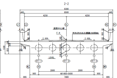
(P7~A2間)
