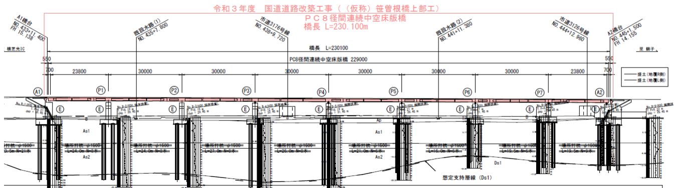
側面図
