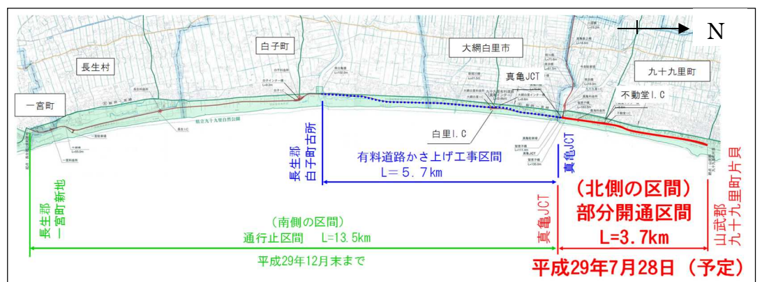
平面図
